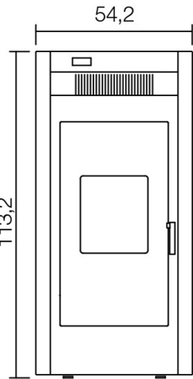
vista fronte stufa
